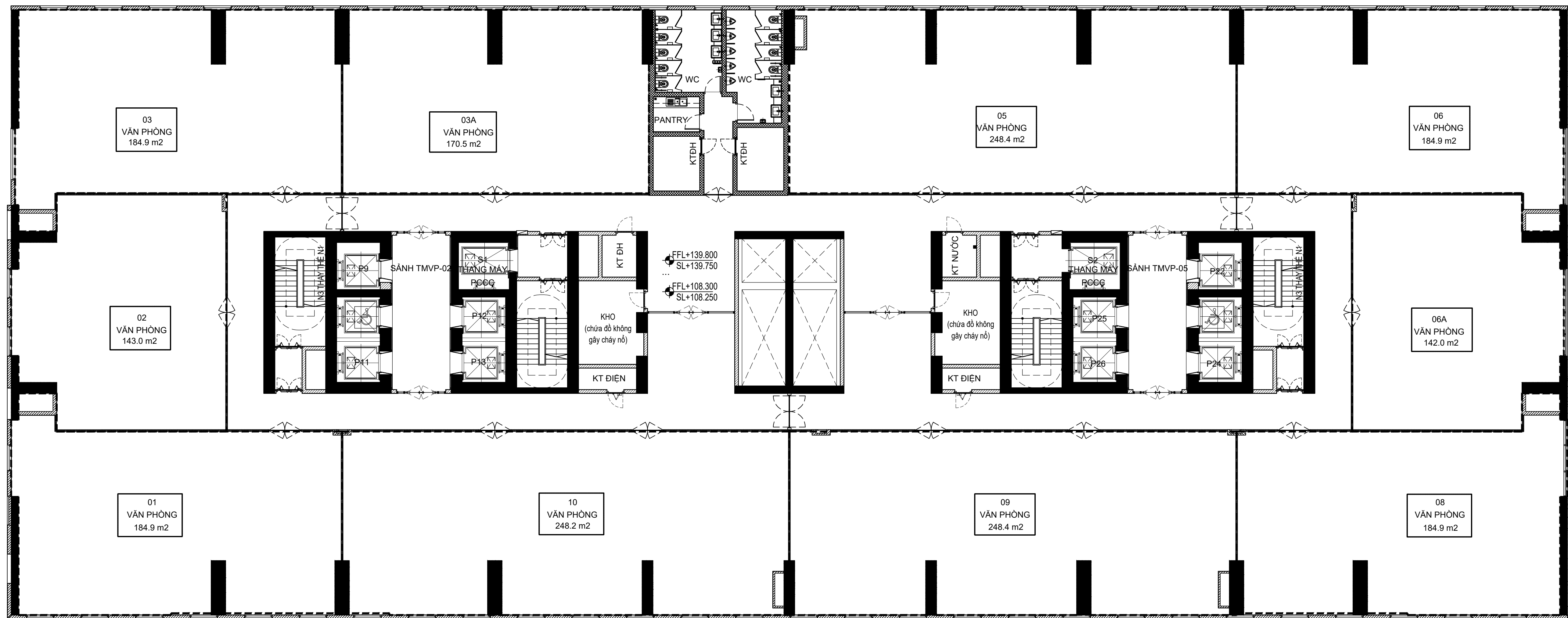
MẶT BẰNG TẦNG 29 - TẦNG 40
